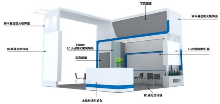
施工材料图 (单位: mm) 所有材料防火等级均达到B1级
